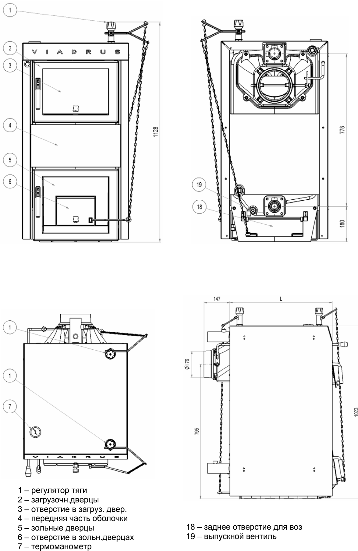
Рис. 36) Схема котла VIADRUS HERCULES U 26 8 – 10 сек.
