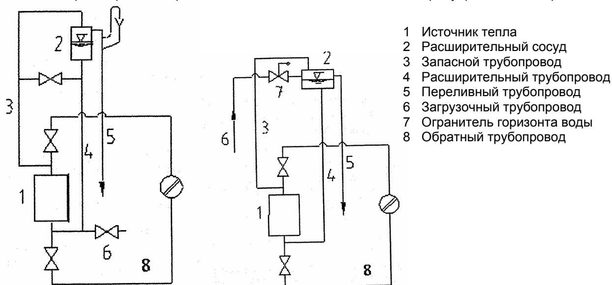
Рис. 8 Образцы подключения открытых расширительных сосудов
