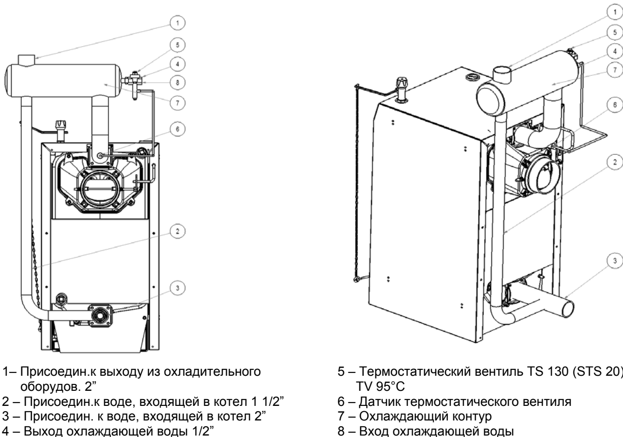
Рис. 4 Охлаждающий контур только для версии с 3 – 7 секциями.
