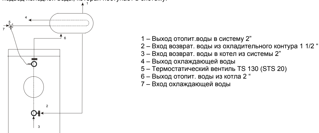
Рис. 5 Гидравлическая схема присоединения охлаждающего контура
