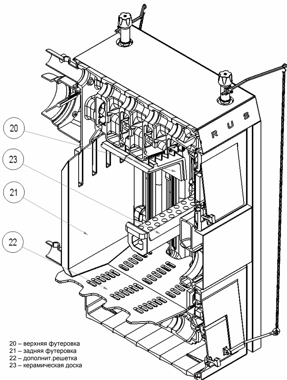
Рис. 3с) Схема котла VIADRUS HERCULES U 26 -расположение дополнительного оснащения
