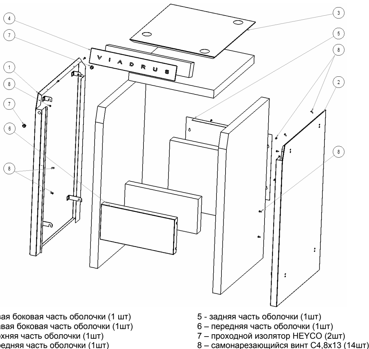
Рис. 10 Установка оболочек котла
