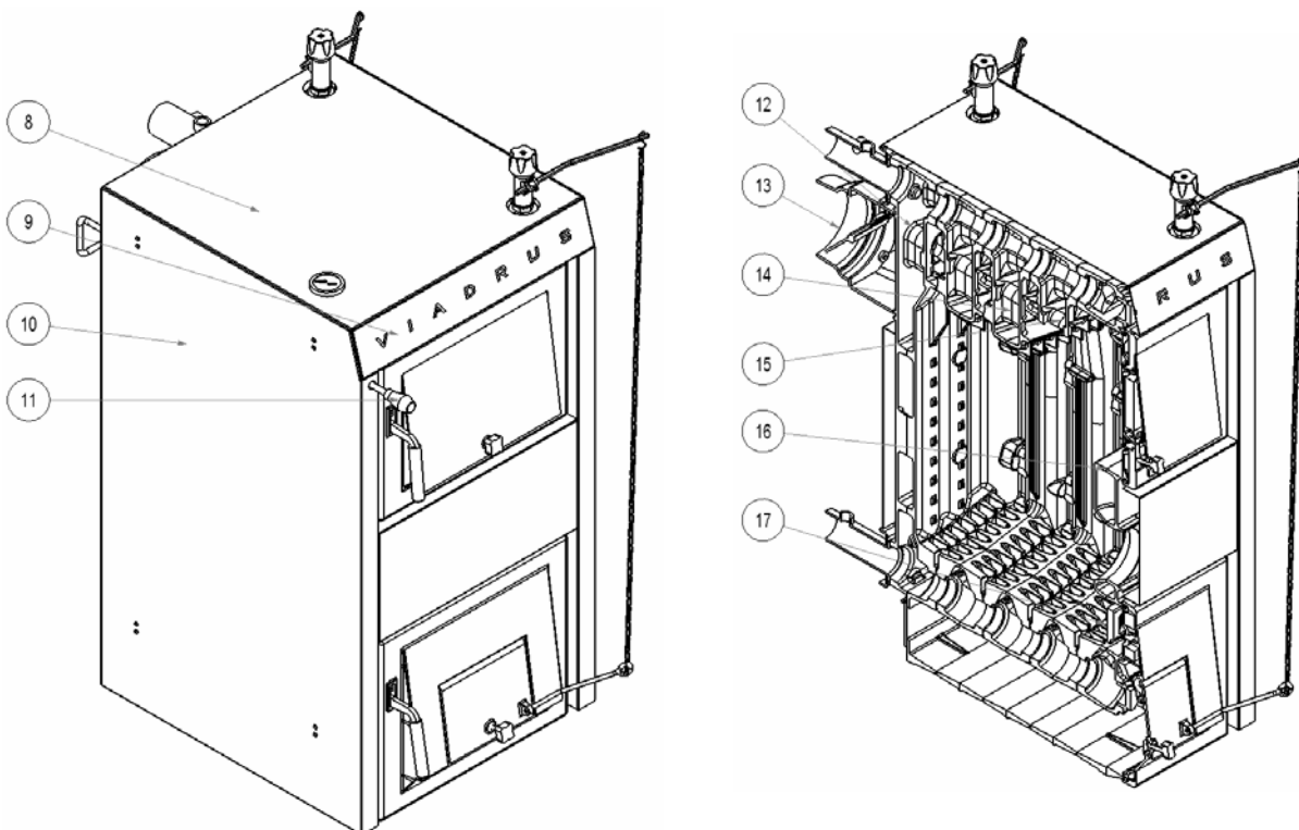
Рис. 3а) Схема котла VIADRUS HERCULES U 26 3 – 7 секций
