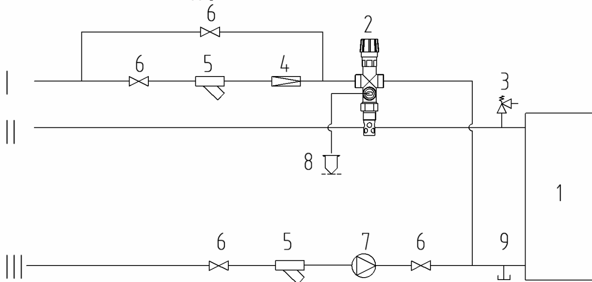
Рис. 6 Двухходовой защитный клапан DBV 1 - 02
