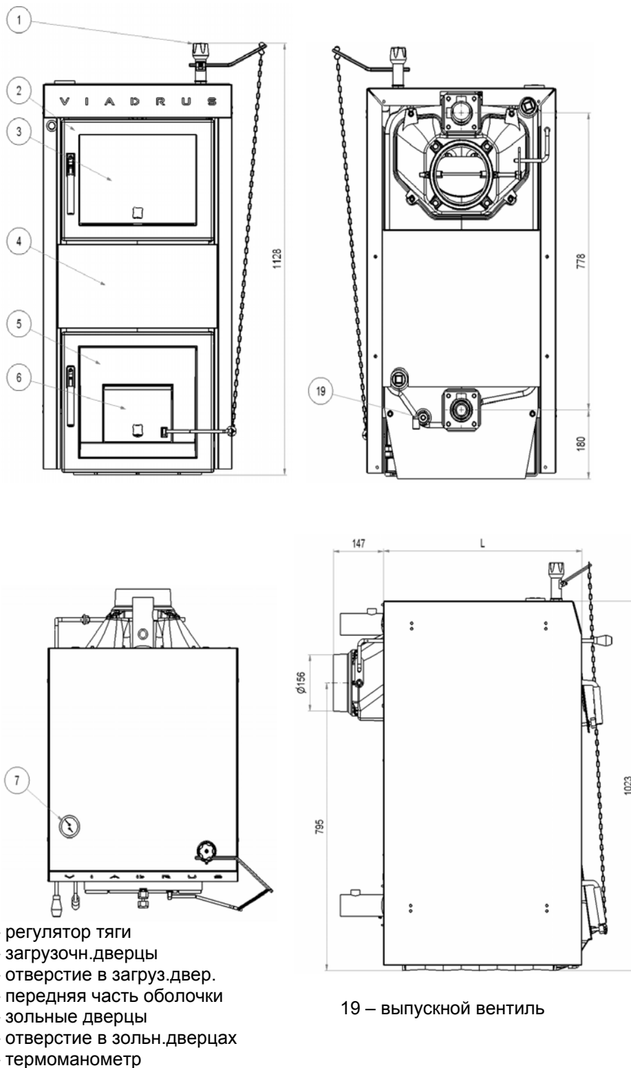
Рис. 2а) Схема котла VIADRUS HERCULES U 26 3 – 7 секций
