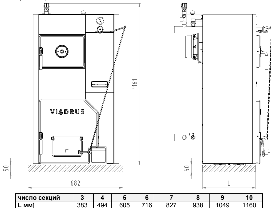
Рис. 5 Размеры цоколя
