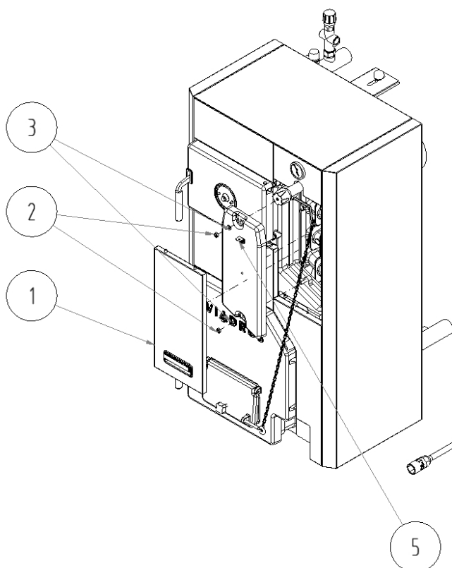
Рис. 13 Демонтаж крышки отверстия для чистки
