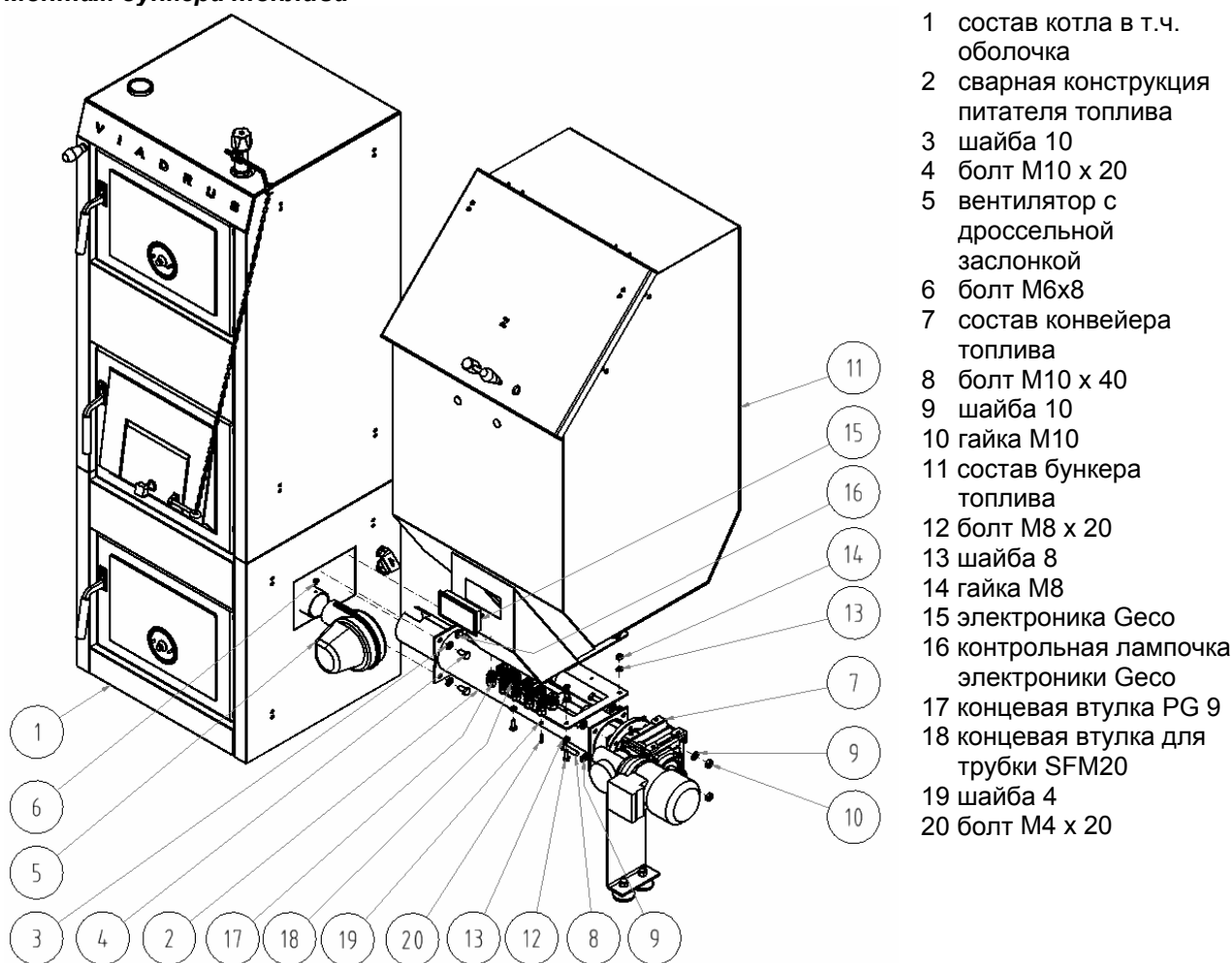
Рис. 10 Монтаж питателя топлива и бункера к котлу
