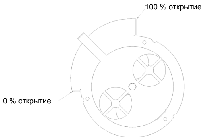
Рис. 14 Дроссельная заслонка вентилятора
