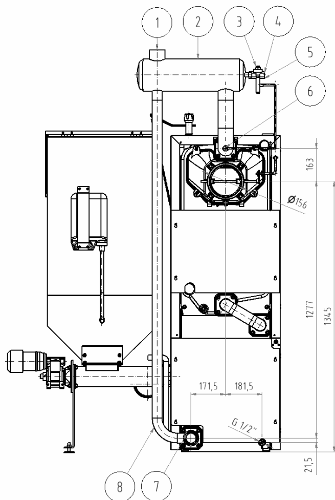
Рис. 3 Охлаждающий контур
