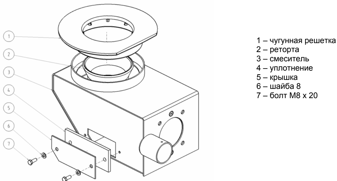
Рис. 2 Горелка с смесителем
