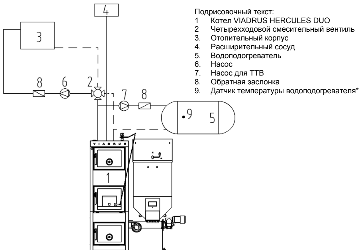
Рис. 11 Блок-схема установки ЦО в системе с четырехходовым вентилем
