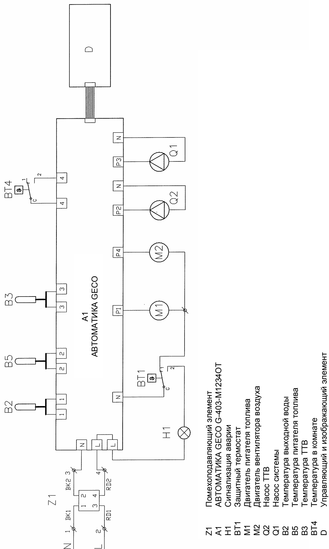
Рис. 12 Блок-схема оборудования и датчиков к регулятору G-403-P02
