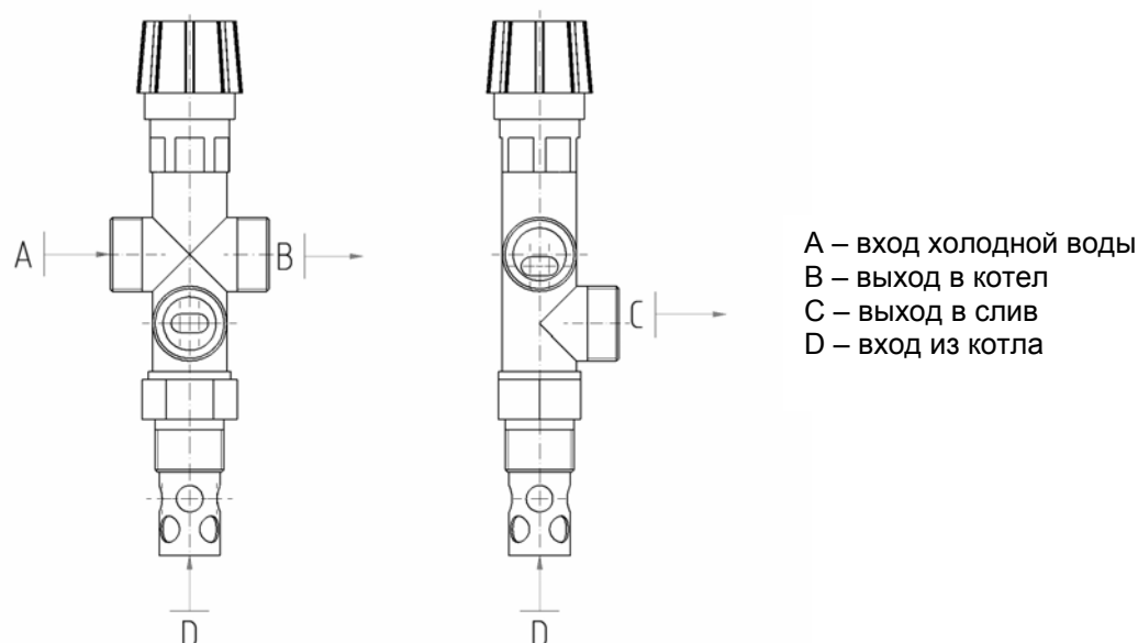
Рис. 5 Двухходовой защитный клапан DVB 1 - 02
