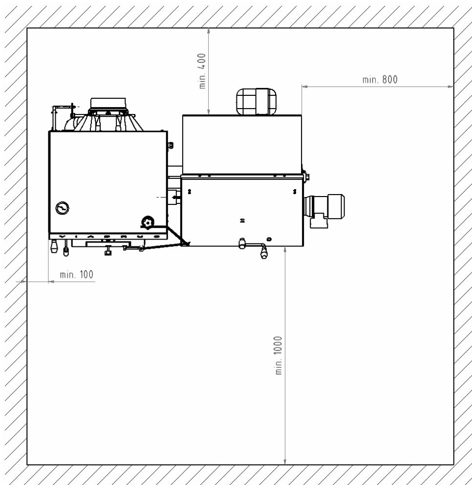
Рис. 8 Расположение котла VIADRUS HERCULES DUO в котельной
