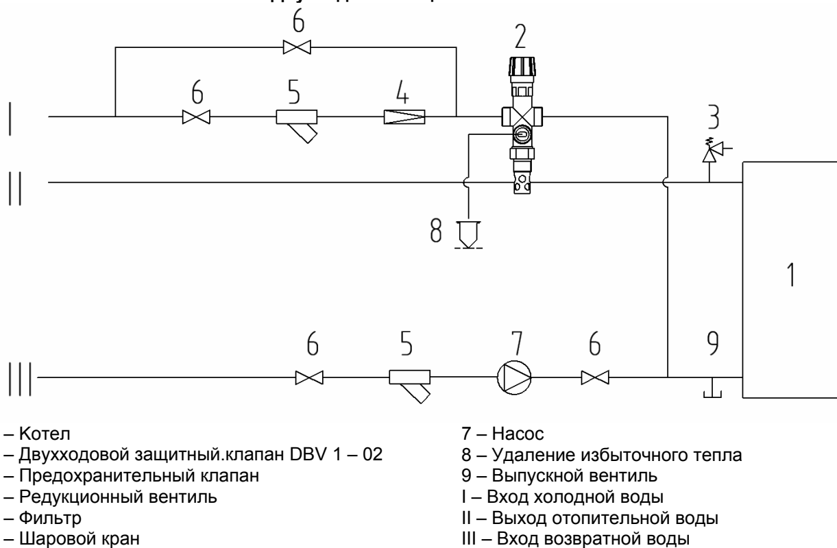
Рис. 6 Рекомендуемая схема включения двухходового защитного клапана DVB 1 - 02
